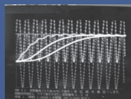
直流・交流二電源回路を ラプラス変換法で解いた例
