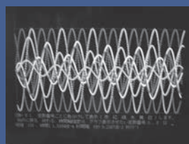
三相交流不平衡負荷回路を ラプラス変換法で解いた例
